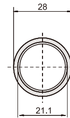
413529 材質: 真鍮 クロームめっき
