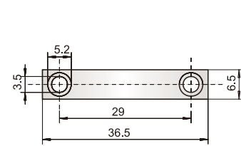
434980 材質: スチール ニッケルめっき
