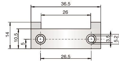
434981 材質: スチール ニッケルめっき
