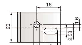
434980 材質: スチール ニッケルめっき
